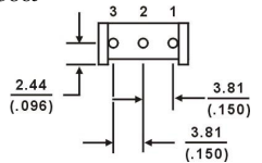
TSR-3386S
